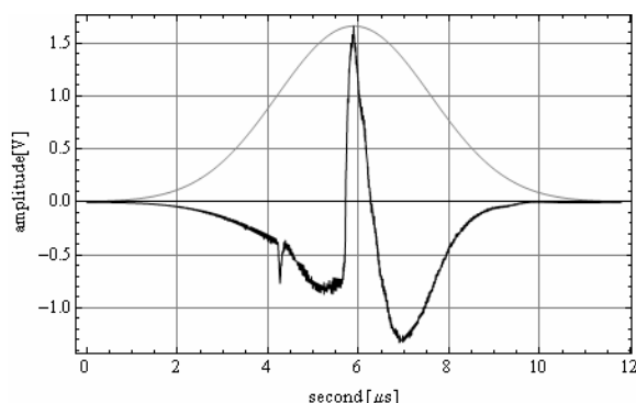
Rys. 3. Sygnał w dziedzinie czasu przeskalowany oknem gaussowskim
