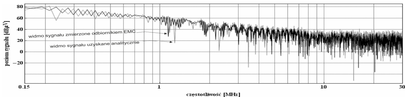
Rys. 4. Widmo częstotliwościowe sygnału zmierzone odbiornikiem EMC oraz uzyskane analitycznie
