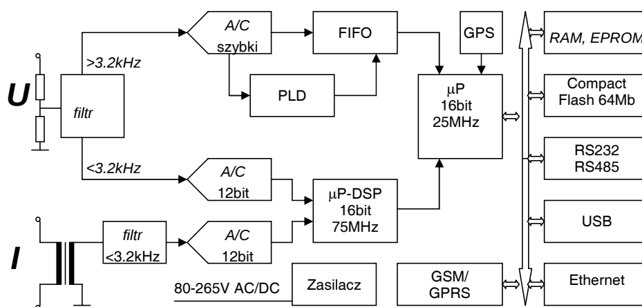
Rys. 3. Struktura analizatora do pomiaru parametrów sieci energetycznej
