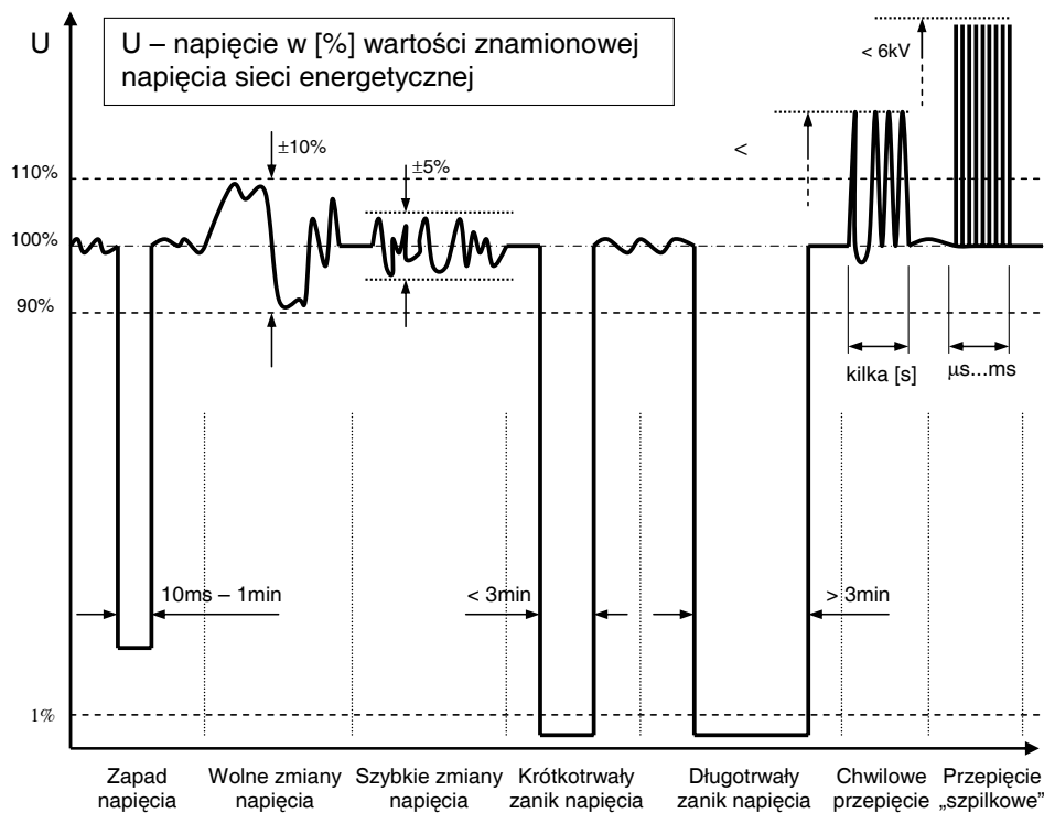
Rys. 1. Parametry opisujące zmiany napięcia w sieci energetycznej
