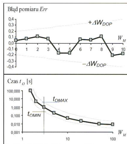
Rys. 2. Charakterystyki badanych urządzeń Fig. 2. Characteristics of equipment under test EUT
