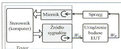
Rys. 1. System do badania urządzeń elektrycznych Fig. 1. System for testing of electrical equipment
