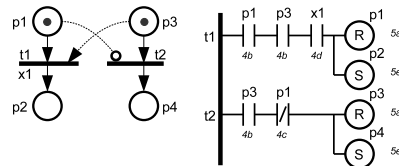
Rys. 2. Realizacja łuków zezwalających i zabraniających
