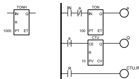
Rys. 9. Realizacja układu czasowego z pamięcią Fig. 9. An implementation of a timer with a memory
