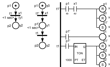
Rys. 4. Realizacja akcji czasowej związanej z tranzycją
