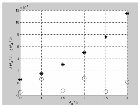
Rys. 2. 'o' – Względne obciążenie estymatora \delta(A_d/q) oraz '*' – względną niepewność standardową typu A \xi(A_d/q) funkcji autokorelacji sygnału harmonicznego z ditherem o rozkładzie równomiernym w funkcji A_d/q , uzyskane z wirtualnego korelatora, przetwornik 6-bitowy
