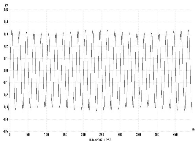
Rys. 5. Wartość wielkości wyjściowej generowana na zaciskach wyjściowych kalibratora Fig. 5. The output setting value generated at the output of calibrator
