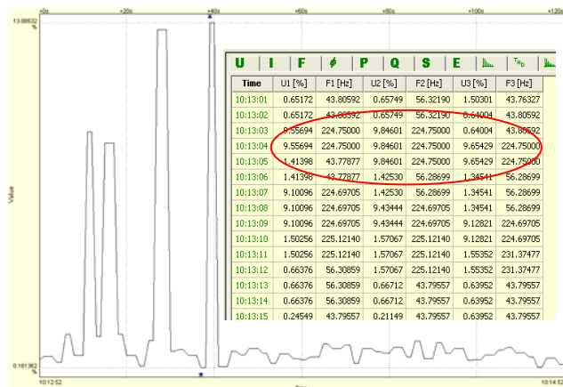
Rys.4. Rezultaty pomiarów napięcia sygnałowego 227Hz. Fig. 4. Results of mains signaling with frequency 227Hz.
