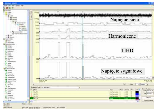
Rys.5. Wyniki rejestracji TIHD i napięcia sygnałowego. Fig. 5. Results of TIHD and mains signaling recording.
