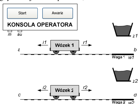
Rys. 1. Schemat przykładowego procesu technologicznego Fig. 1. Case study of technological discrete process
