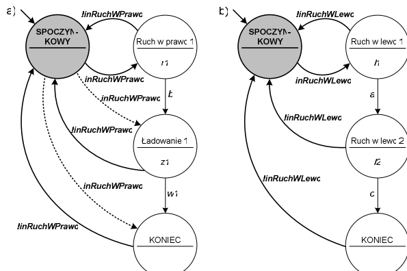
Rys. 4. Wybrane automaty FSM z dodatkowymi przejściami i stanami bezczynności Fig. 4. Some of FSMs with additional special transitions and idle states
