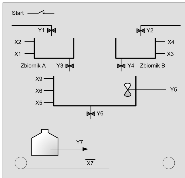
Rys. 2. Przykład procesu przemysłowego Fig. 2. Example of manufacturer process
