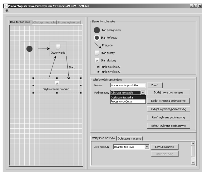
Rys. 1. Okno główne edytora graficznego Fig. 1. The graphics editor main window
