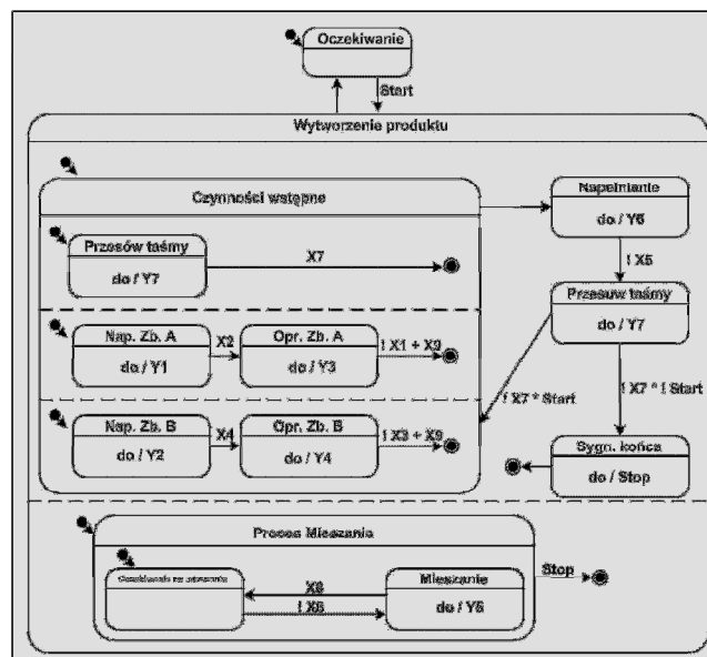
Rys. 5. Zmodyfikowany diagram maszyny stanów UML Fig. 5. Modified UML state machine diagram
