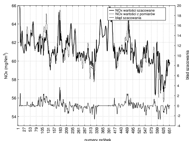
Rys. 4. Przebieg oryginalnej zmiennej \text{NO}_x oraz jej estymacja
