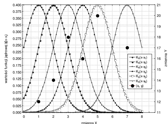
Rys. 3. Jądrowy estymator funkcji regresji: przebiegi funkcji jądrowej Fig. 3. Kernel estimator of regression function: kernel function plots
