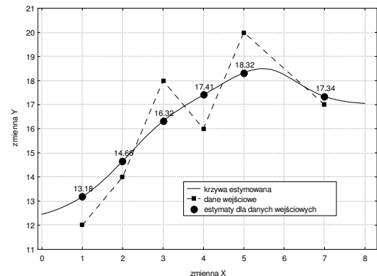
Rys. 2. Jądrowy estymator funkcji regresji: wyniki estymacji Fig. 2. Kernel estimator of regression function: estimation results
