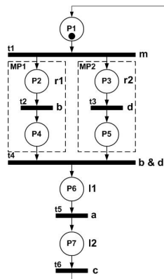
Rys. 8. Sieć Petriego dla omawianego przykładu Fig. 8. Petri net for discussed example
