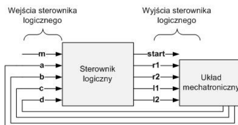
Rys. 3. Sterownik logiczny
