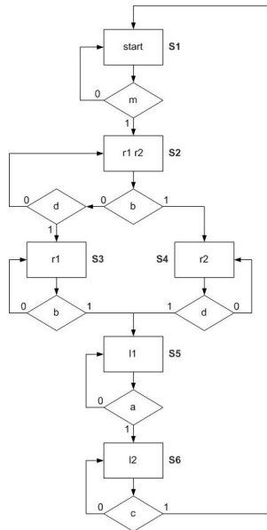
Rys. 4. Algorytm procesu sterowania dla badanego przykładu przedstawiony za pomocą algorytmicznej maszyny stanów
